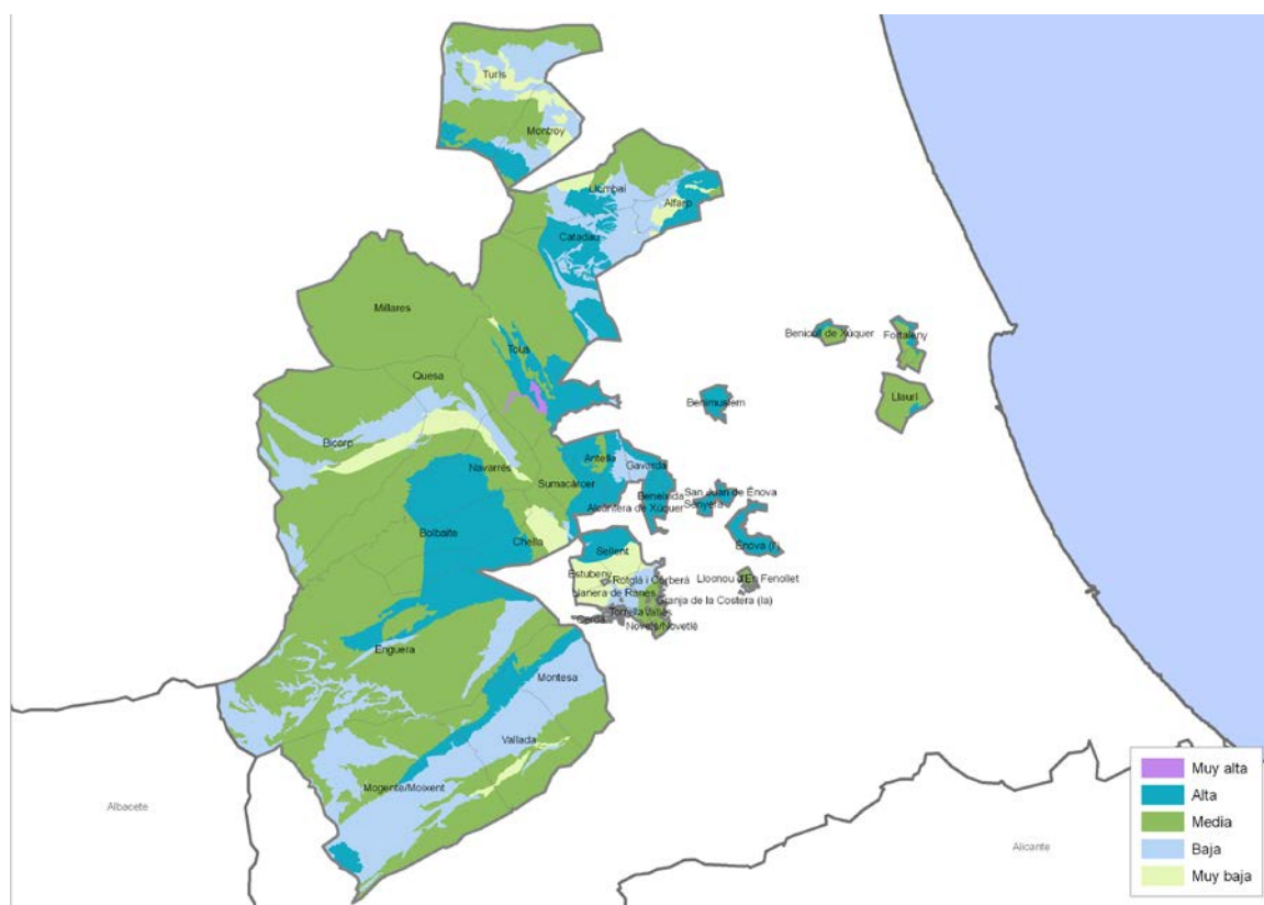
Mapa 8 Vulnerabilidad de los acuíferos en el territorio del GAL
