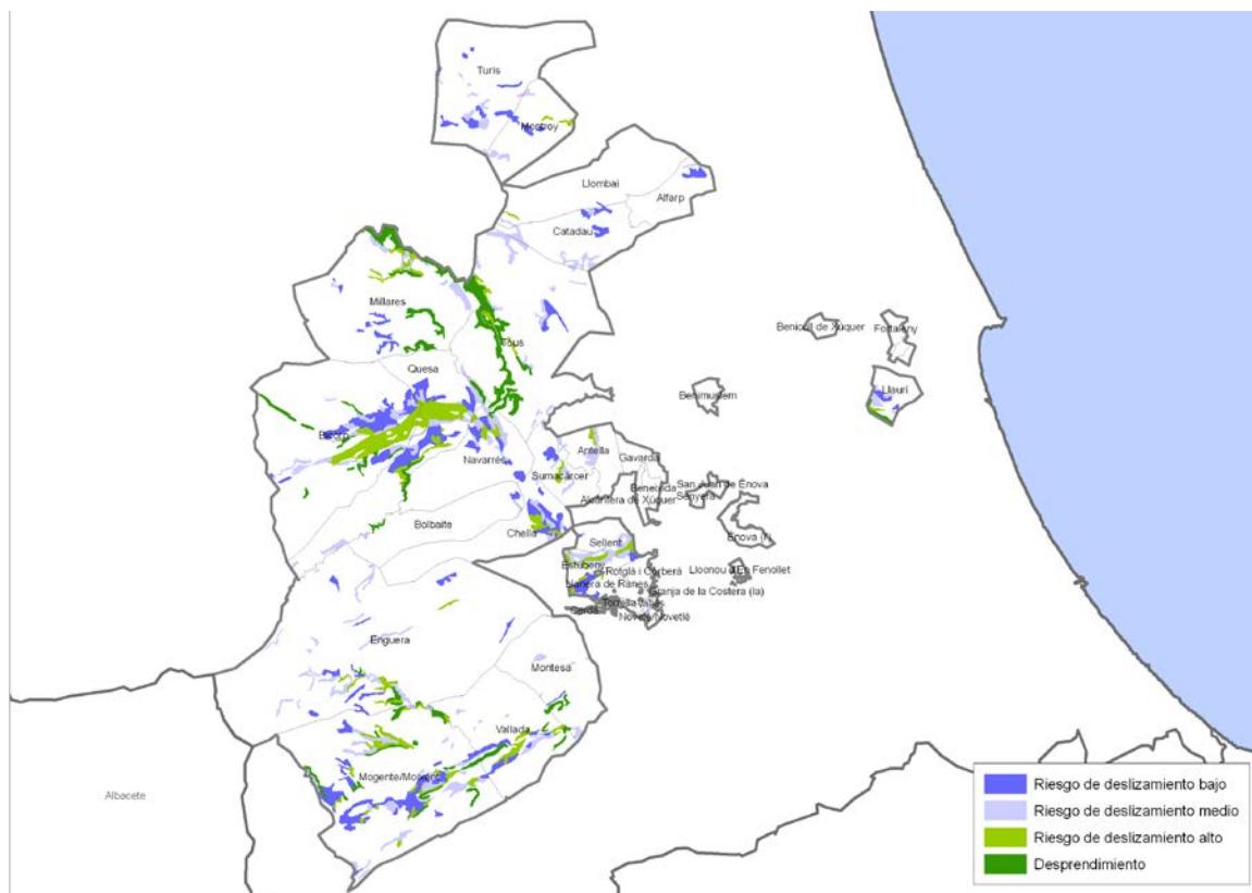
Mapa 6 Riesgo de deslizamiento en el territorio del GAL
