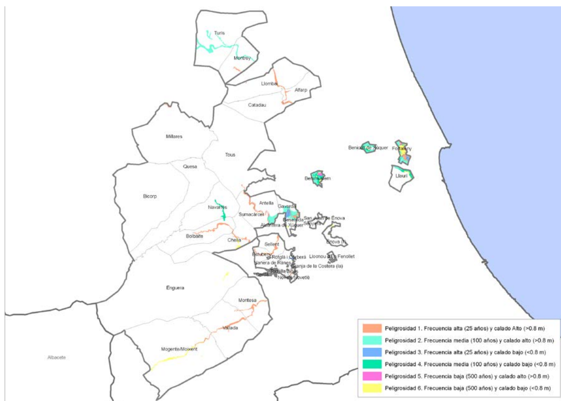
Mapa 9 Riesgo de inundación en el territorio del GAL
